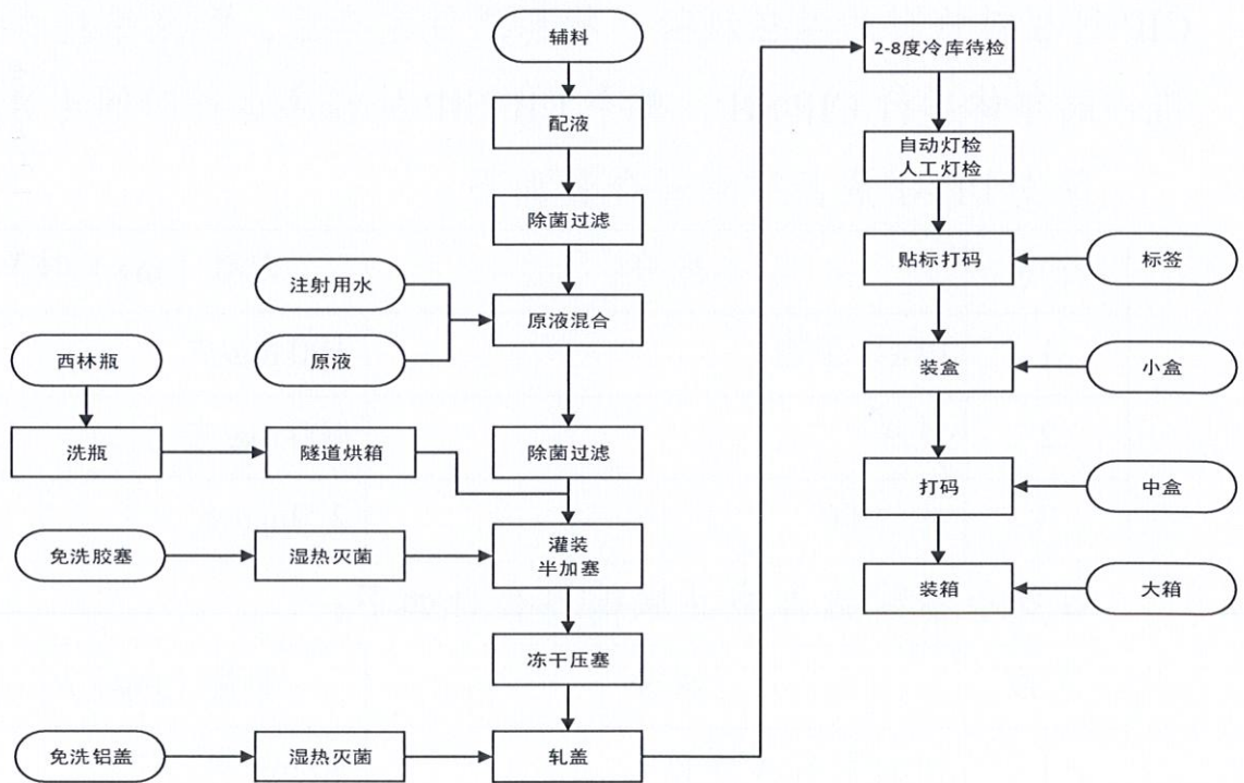
图 1. PD-1 工艺方框流程图
